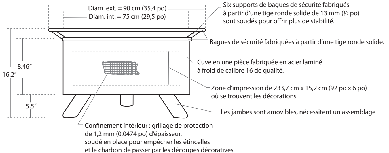
GRILLAGE DE PROTECTION
